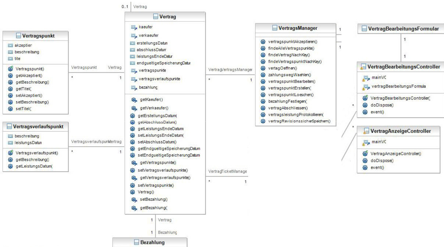
UML-Diagramm für ‚Vertrag‘
