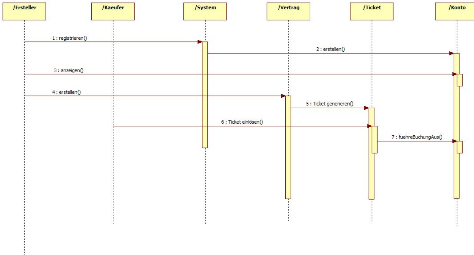
Sequenzdiagramm für 'Ticket' und 'Konto'
